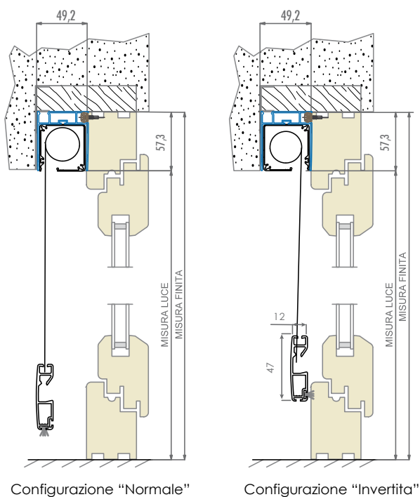
sez A-A
