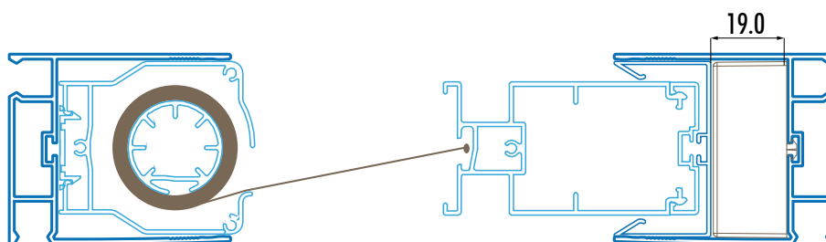
Predisposizione con zanzariera in versione "Standard": con zanzariera e profilo di riscontro con spessori di 19 mm
