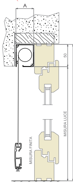
Configurazione "Normale"
