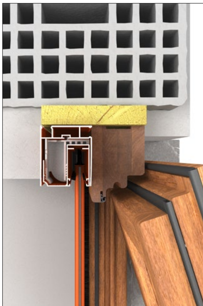
Configurazione "Invertita"
