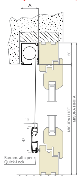
Configurazione "Invertita" barramaniglia Alta
