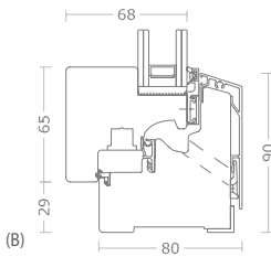
B - Nodo Inferiore con traverso
