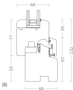
B - Nodo Inferiore con traverso
