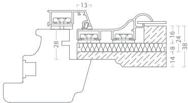
TRAVERSINI SDL tipo CL/CQ 35 mm
