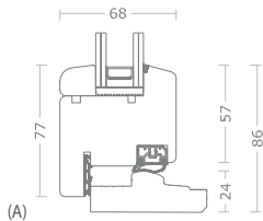
A - Nodo Inferiore con soglia
