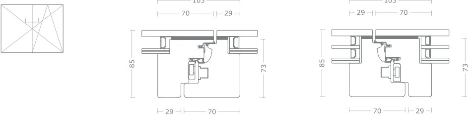
Sezione centrale senza montante aggiunto
