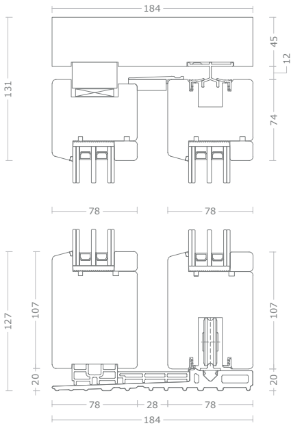
Sezione verticale
