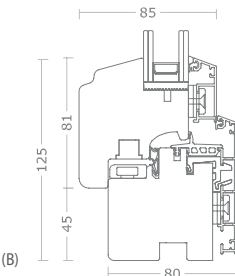
B - Nodo Inferiore con traverso
