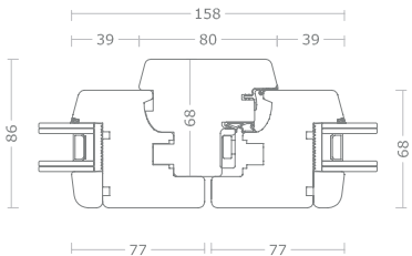
Sezione centrale con montante aggiunto
