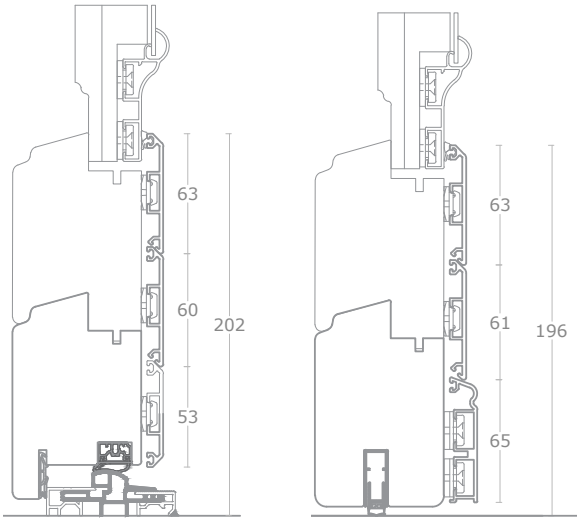
Nodo inferiore
