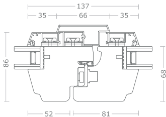
Sezione centrale senza montante aggiunto
