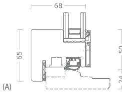
A - Nodo Inferiore con soglia
