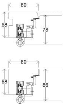
Nodo laterale
