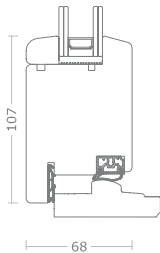
Traverso inferiore 107
