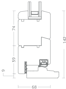
N° 1 zoccolo aggiuntivo; profilo anta da 77 mm
