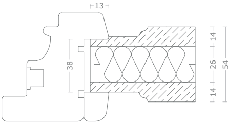
Sezione 78
