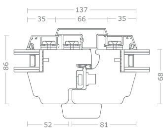
Sezione centrale senza montante aggiunto con maniglia centrale
