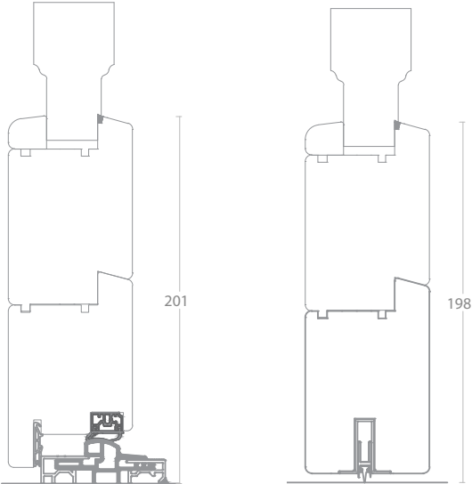
Nodo inferiore
