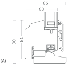
A - Nodo Inferiore con soglia
