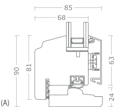
A - Nodo Inferiore con soglia
