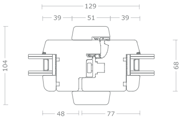
Sezione centrale senza montante aggiunto con maniglia centrale
