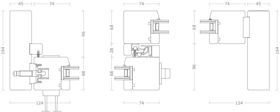
Sezione orizzontale
