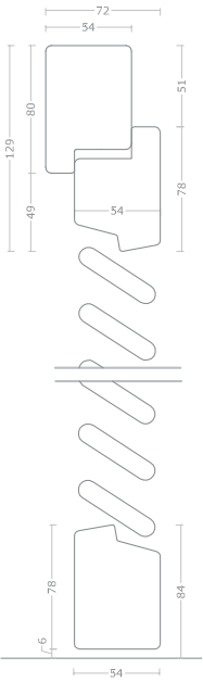
Lamella fissa Fixed louver
