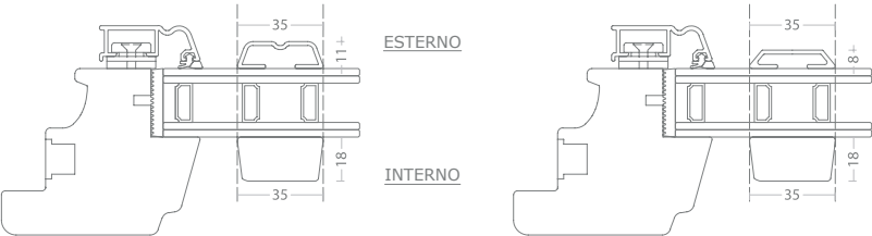
TRAVERSINI SDL tipo CL/CL 35 mm
