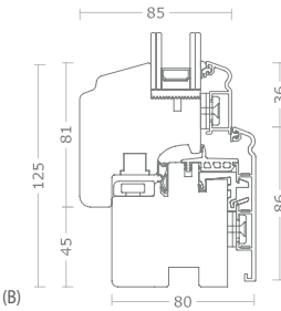
B - Nodo Inferiore con traverso
