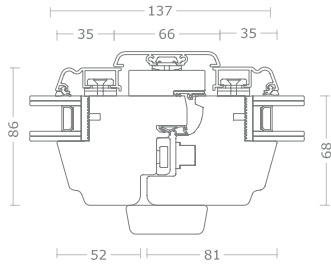
Sezione centrale senza montante aggiunto con maniglia centrale
