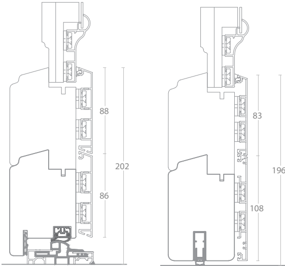
Nodo inferiore
