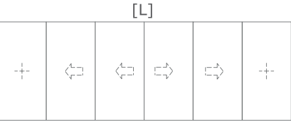
6 ante 4 ante scorrevoli + 2 fissi laterali
