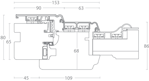
Nodo laterale - superiore
