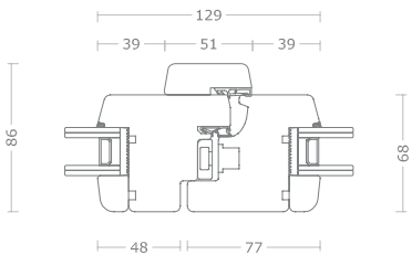
Sezione centrale senza montante aggiunto
