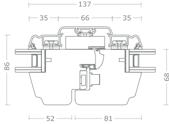
Sezione centrale senza montante aggiunto
