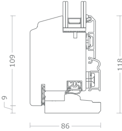
N° 1 profilo anta da 109 mm Altezza totale = 118 mm
