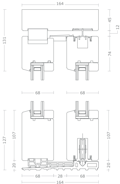
Sezione verticale
