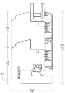
N° 1 zoccolo aggiuntivo da 81 mm; profilo anta da 81 mm
