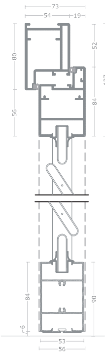
Lamella fissa Fixed louver
