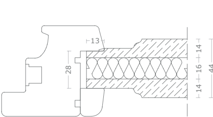
Sezione 68
