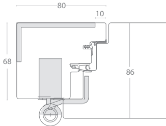
Nodo laterale
