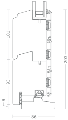
Profilo anta da 109 mm, Opzione N° 1 zoccolo aggiuntivo Altezza totale = 118 mm
