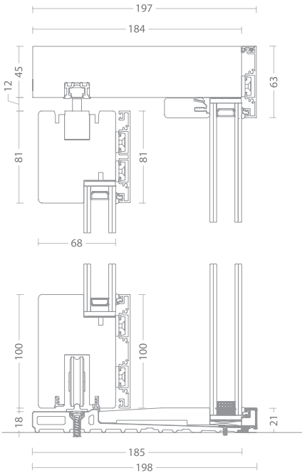
Sezione verticale
