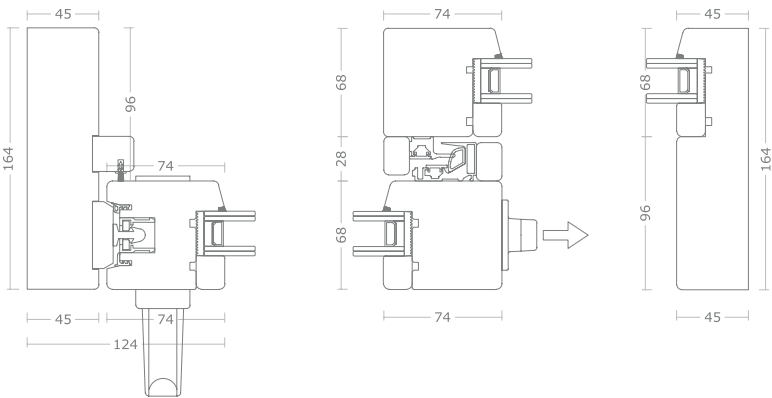
Sezione orizzontale
