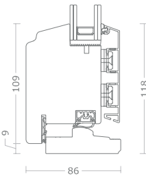
Traverso inferiore 109
